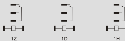
接线图 (底视)
