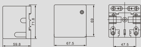
JQX-62FH 1Z: 外形尺寸(导轨型)
