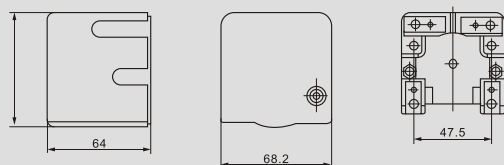
JQX-62FH 1Z: 外形尺寸(导轨型)
